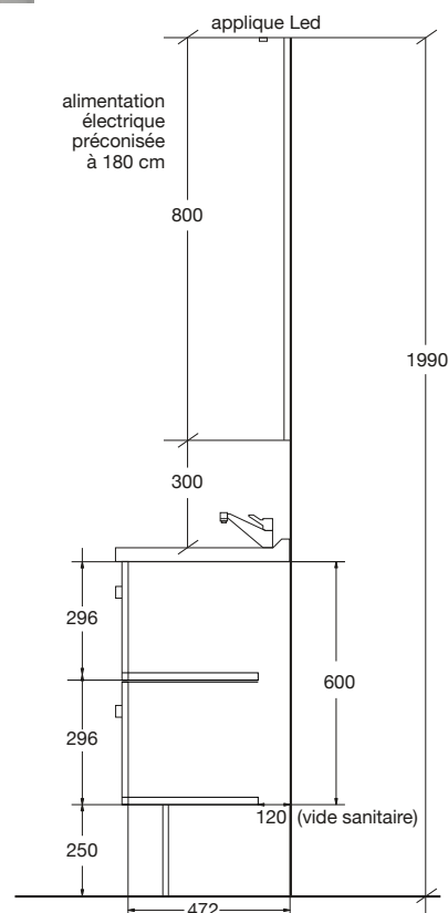
Colonne avec 1 porte miroitée
